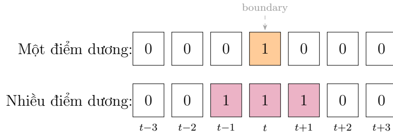
Hình 3.9: Minh họa nhãn một điểm dương (one-hot) và nhiều điểm dương (many-hot). Nhãn một điểm dương chỉ gán 1 tại đúng khung ranh giới t ; nhãn nhiều điểm dương mở rộng thêm t \pm 1 , cung cấp tín hiệu gradient dày đặc hơn quanh vùng ranh giới.
