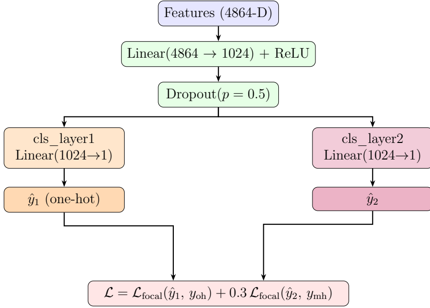
Hình 3.8: Kiến trúc tầng phân loại (ClassificationHead) trong AutoShotV2. Tầng phân loại này nhận đặc trưng 4864-D từ mạng xương sống (đóng băng) và sinh hai đầu ra song song: nhánh một điểm dương (one-hot) định vị ranh giới chính xác và nhánh nhiều điểm dương (many-hot) học ngữ cảnh vùng biên.
