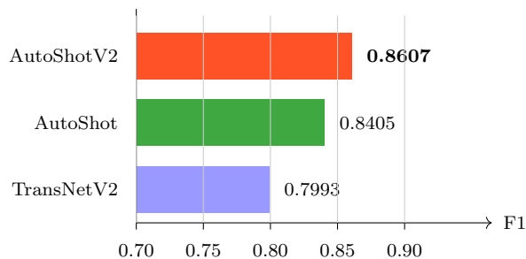
Hình 4.3: So sánh F1 giữa các mô hình trên tập SHOT (200 video kiểm tra). AutoShotV2 đạt F1 = 0.8607 theo lựa chọn tốt nhất trong protocol so sánh chính, cải thiện +2.02 điểm phần trăm so với AutoShot tự chạy lại và +6.14 điểm phần trăm so với TransNetV2 mô hình cơ sở.
