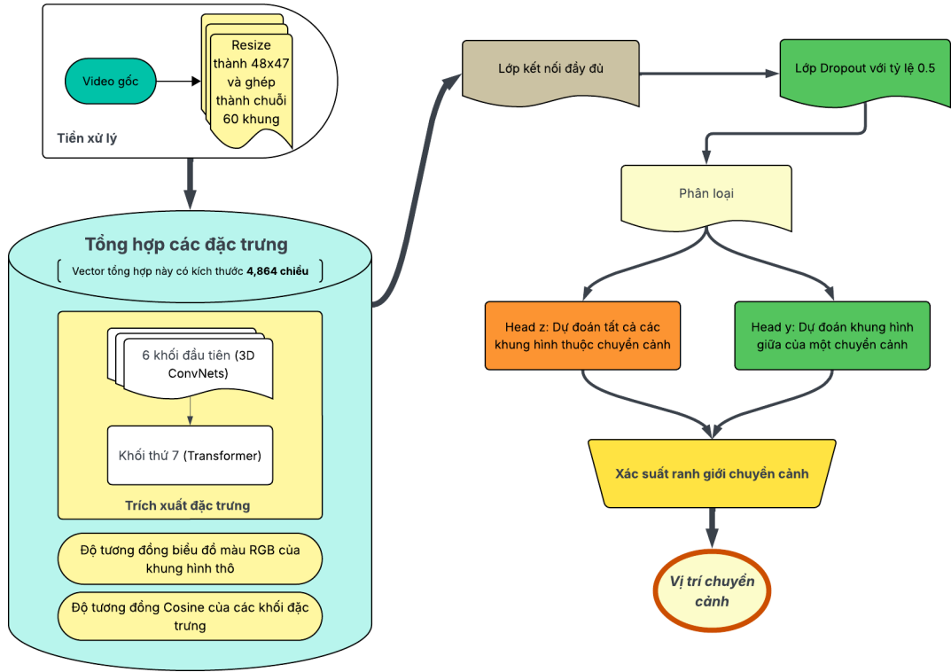
Hình 3.1: Sơ đồ luồng xử lý tổng quan của hệ thống phát hiện ranh giới cảnh quay AutoShot/AutoShotV2. Video đầu vào trải qua bước tiền xử lý, trích xuất đặc trưng kết hợp với nhánh tính độ tương đồng để tạo vector đặc trưng tổng hợp 4864-chiều, sau đó qua các lớp kết nối đầy đủ và phân loại song song để dự đoán xác suất ranh giới.
