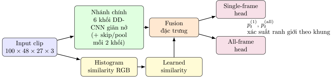
Hình 3.3: Tổng quan kiến trúc TransNetV2: 6 khối DDCNN giãn nở xếp chồng (nhánh chính) kết hợp với nhánh đặc trưng tương đồng (histogram RGB + learned similarity), đầu ra qua hai đầu phân loại song song (single-frame head và all-frame head). Kết nối tắt và pooling trung bình không gian được áp dụng sau mỗi hai khối DDCNN.
