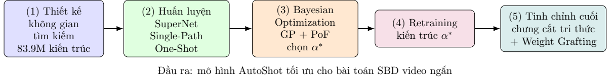
Hình 3.7: Sơ đồ 5 pha của quy trình NAS trong AutoShot: (1) Thiết kế không gian tìm kiếm với 83.9M kiến trúc; (2) Huấn luyện SuperNet theo chiến lược Single-Path One-Shot; (3) Tìm kiếm kiến trúc tối ưu bằng Bayesian Optimization (GP + PoF); (4) Huấn luyện lại kiến trúc \alpha^* ; (5) Tinh chỉnh bằng chưng cất tri thức và Weight Grafting.
