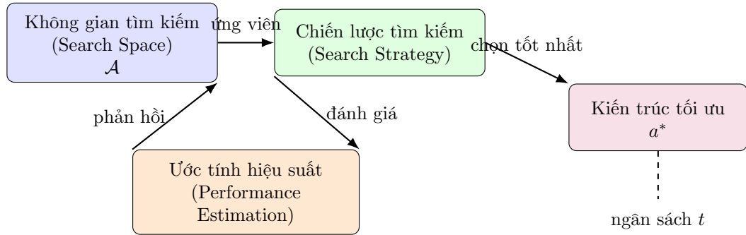
Hình 3.2: Sơ đồ ba thành phần cốt lõi của NAS: không gian tìm kiếm (không gian tìm kiếm), chiến lược tìm kiếm (search strategy) và chiến lược ước tính hiệu suất (performance estimation strategy) liên kết nhau thành vòng lặp phản hồi. Đầu ra là kiến trúc tối ưu a^* đáp ứng ngân sách tính toán t .
