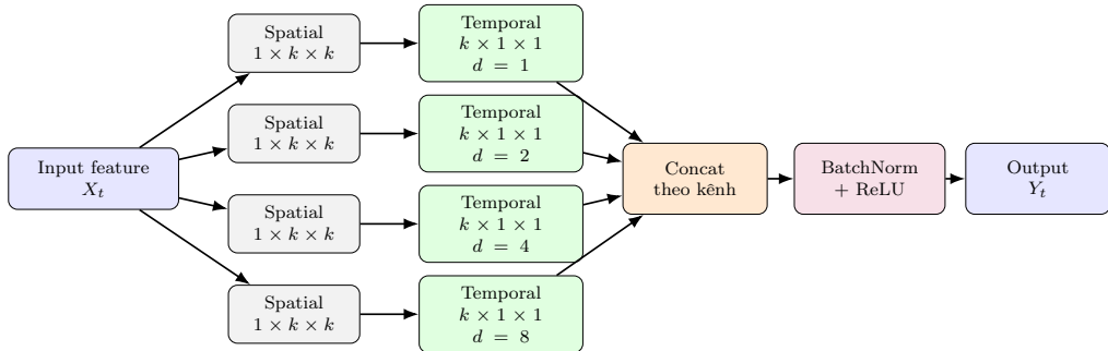
Hình 3.4: Cấu trúc chi tiết của khối DDCNN trong TransNetV2: 4 nhánh tích chập thời gian 1D với độ giãn nở d \in \{1, 2, 4, 8\} song song nhau, đầu ra được nối ghép theo chiều kênh. Mỗi nhánh trước tiên qua tích chập không gian 2D ( 1 \times k \times k ) rồi mới qua tích chập thời gian 1D giãn nở ( k \times 1 \times 1 ).
