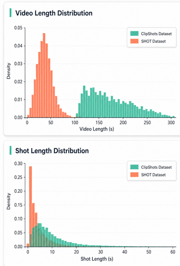
Hình 4.2: Sự phân bố độ dài video (trên) và độ dài shot (dưới). Có thể thấy sự chênh lệch rõ rệt: shot trong SHOT tập trung dày đặc ở vùng dưới 5 giây.
