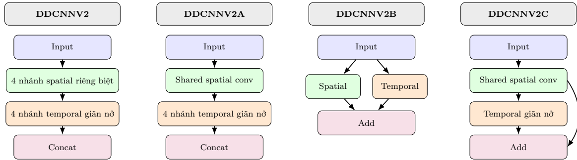
Hình 3.6: Bốn biến thể khối tích chập 3D phân tách trong không gian tìm kiếm của AutoShot. Từ trái qua phải: DDCNNV2 (spatial riêng biệt từng nhánh, concat), DDCNNV2A (shared spatial, concat), DDCNNV2B (spatial + temporal song song, cộng dồn theo P3D), DDCNNV2C (spatial truyền tuần tự vào temporal, cộng dồn). Tất cả đều dùng tích chập thời gian 1D giãn nở đa nhánh.
