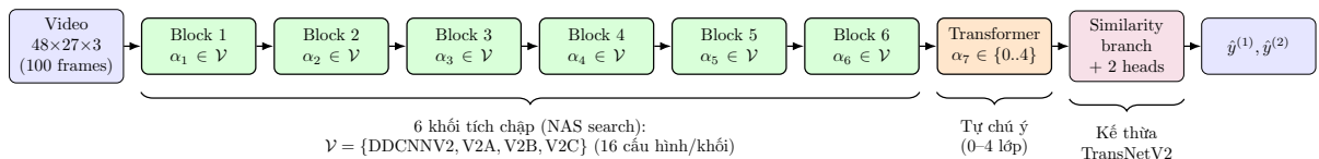
Hình 3.5: Sơ đồ tổng thể mô hình AutoShot gồm 7 vị trí kiến trúc cần tìm kiếm. Sáu vị trí đầu là các khối tích chập phân tách 3D chọn từ \mathcal{V} = \{DDCNNV2, DDCNNV2A, DDCNNV2B, DDCNNV2C\} với các siêu tham số (nc, nd) ; vị trí thứ 7 là khối Transformer 1D với số lớp tự chú ý \alpha_7 \in \{0, 1, 2, 3, 4\} . Nhánh similarity và hai đầu phân loại được kế thừa nguyên vẹn từ TransNetV2, do đó mọi cải thiện đo được đều quy về sự khác biệt ở 7 quyết định \alpha_1, \dots, \alpha_7 của NAS.
