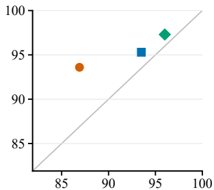
ContextASR-ZH
