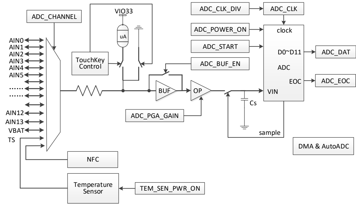
图 15-1 ADC 结构图
