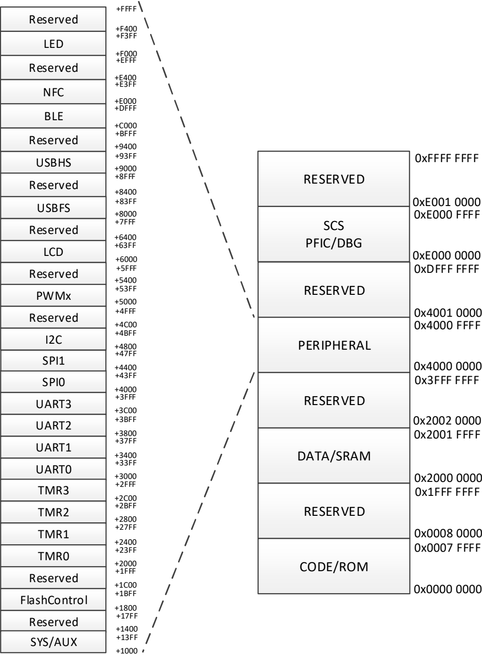
图 2-2 存储器映射图
