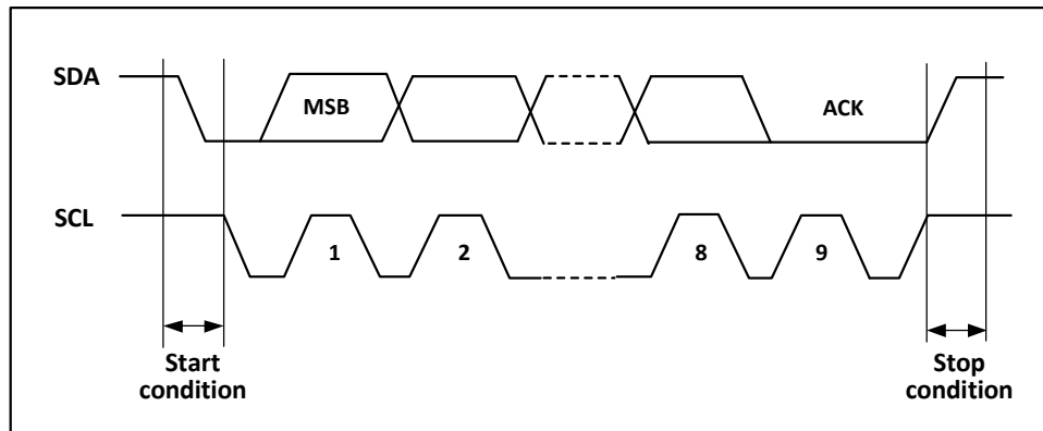
图 12-1 I2C 时序图
