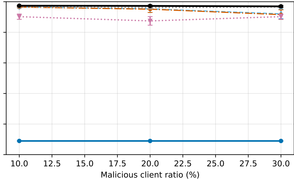
Update-scaling
