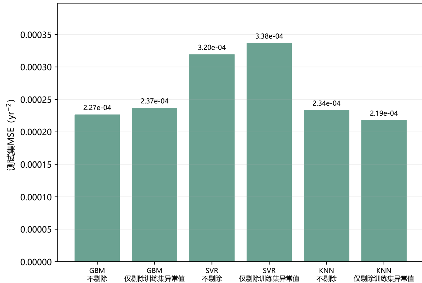
(b) k值预测模型的测试集MSE
