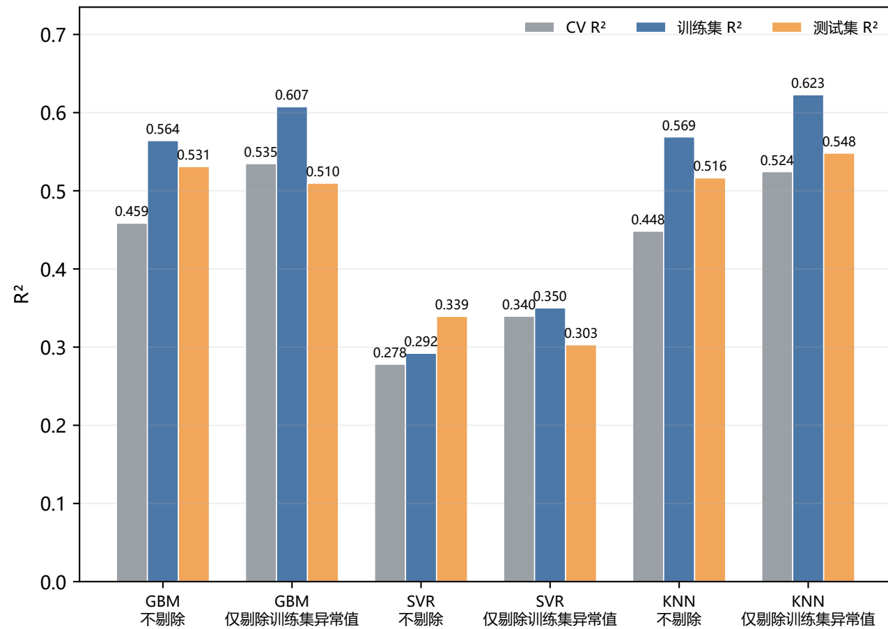
(a) k值预测模型的R 2 比较
