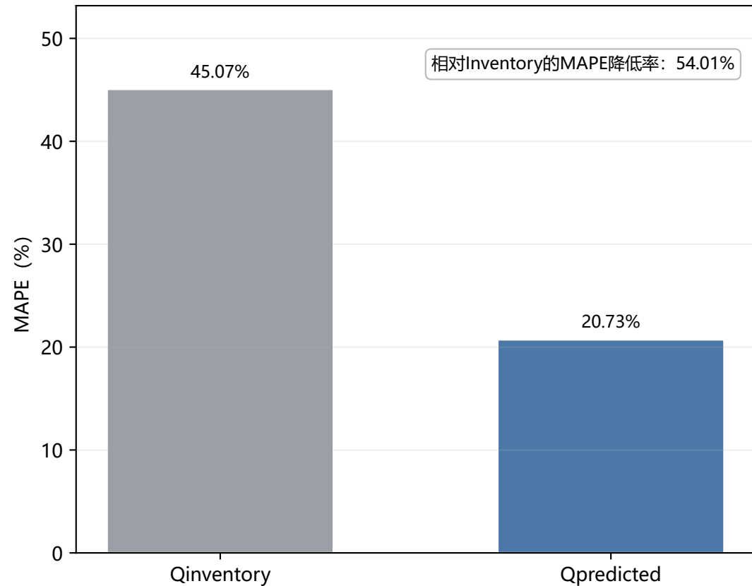
(a) 总体MAPE比较
