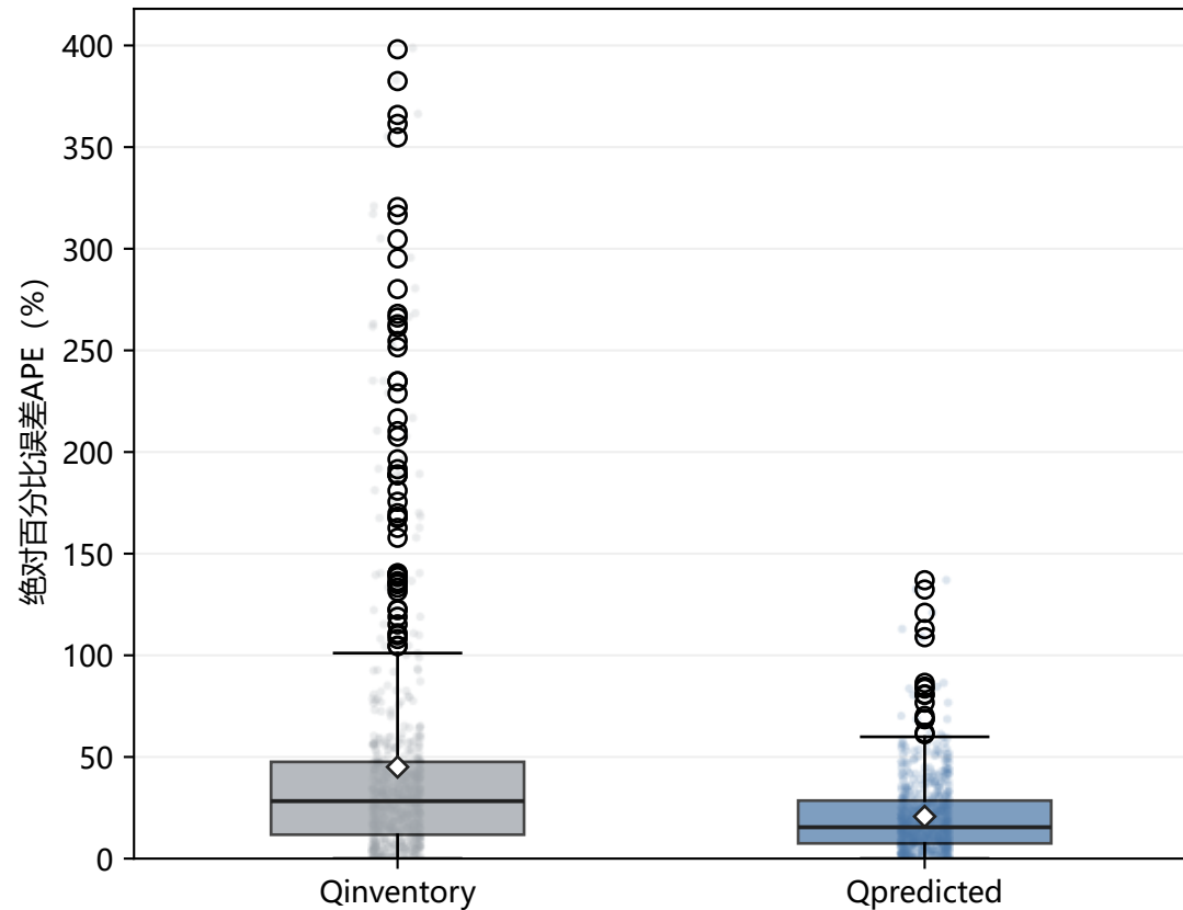
(b) 逐记录APE分布 (n = 550)
