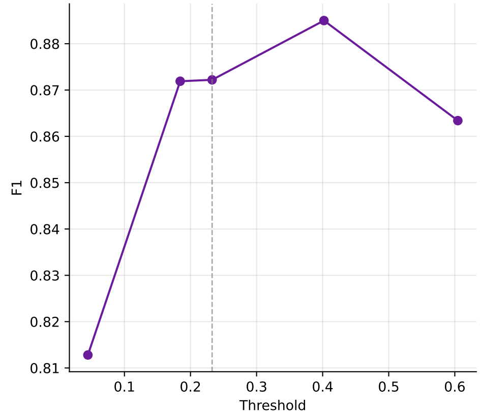
F1 Score
