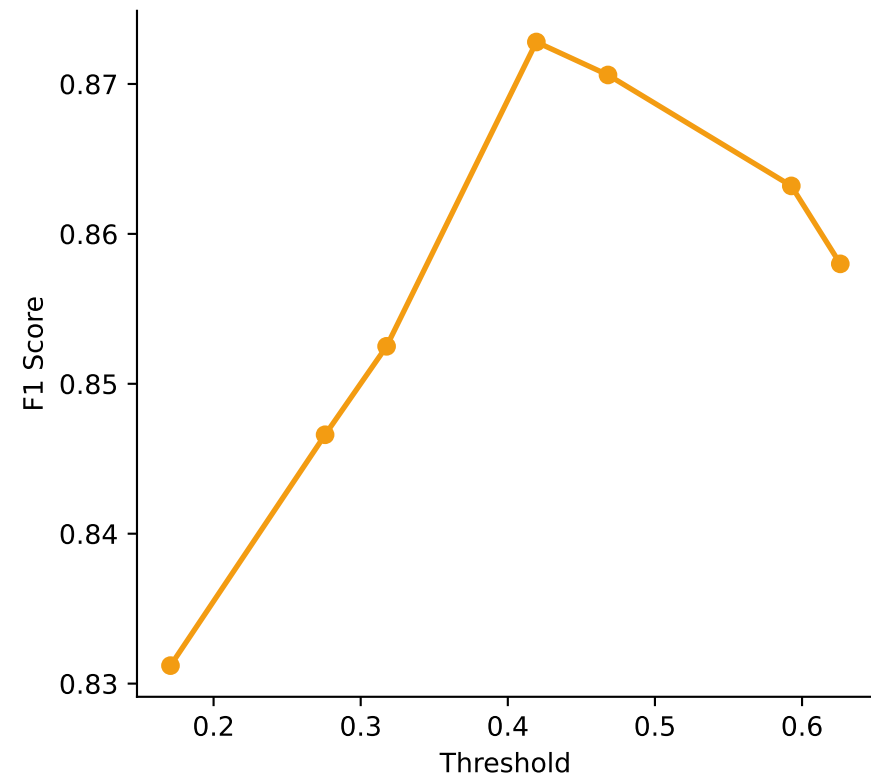
F1 Score
