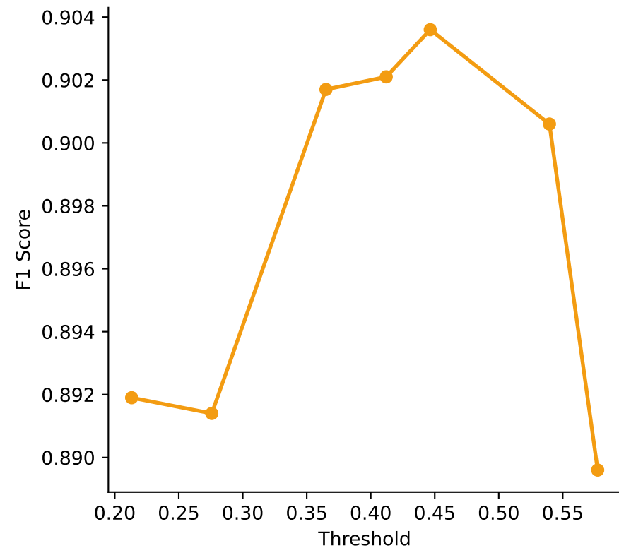
F1 Score
