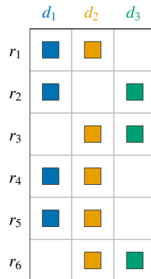
(d) Compressed product JS
