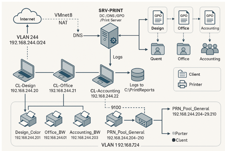
Hình: Sơ đồ cấu trúc tổng thể hệ thống Printer Server
