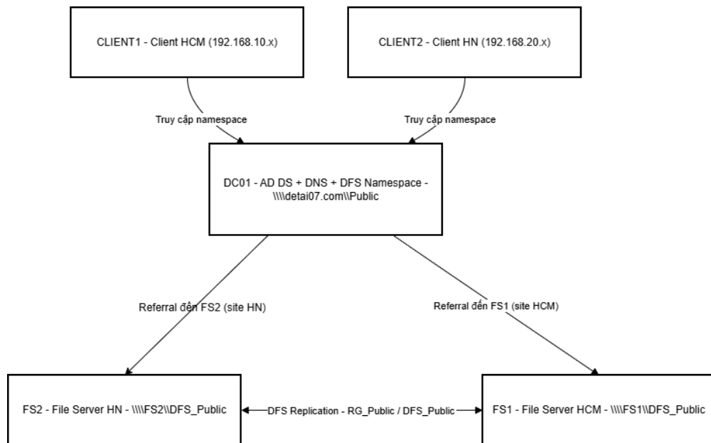
Hình 3.2: Sơ đồ kiến trúc tổng thể hệ thống
