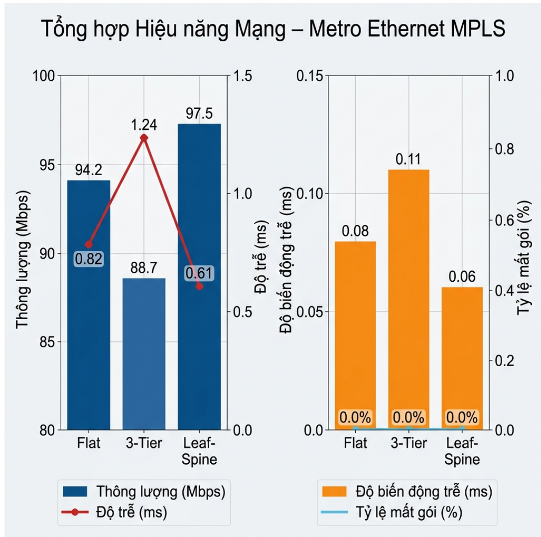
Hình 5.1: Tổng hợp 4 chỉ số hiệu năng: Throughput, Delay, Jitter, Packet Loss theo từng kịch bản
