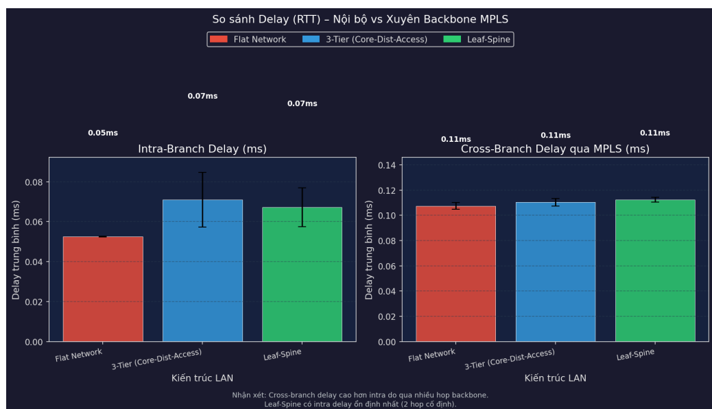
Hình 5.5: So sánh độ trễ (Ping RTT) giữa các kiến trúc – intra và cross-branch
