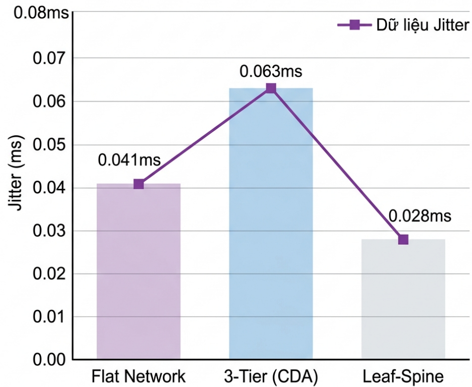
Hình 5.4: Jitter (ms) theo từng kịch bản đo lường – 3 kiến trúc LAN
