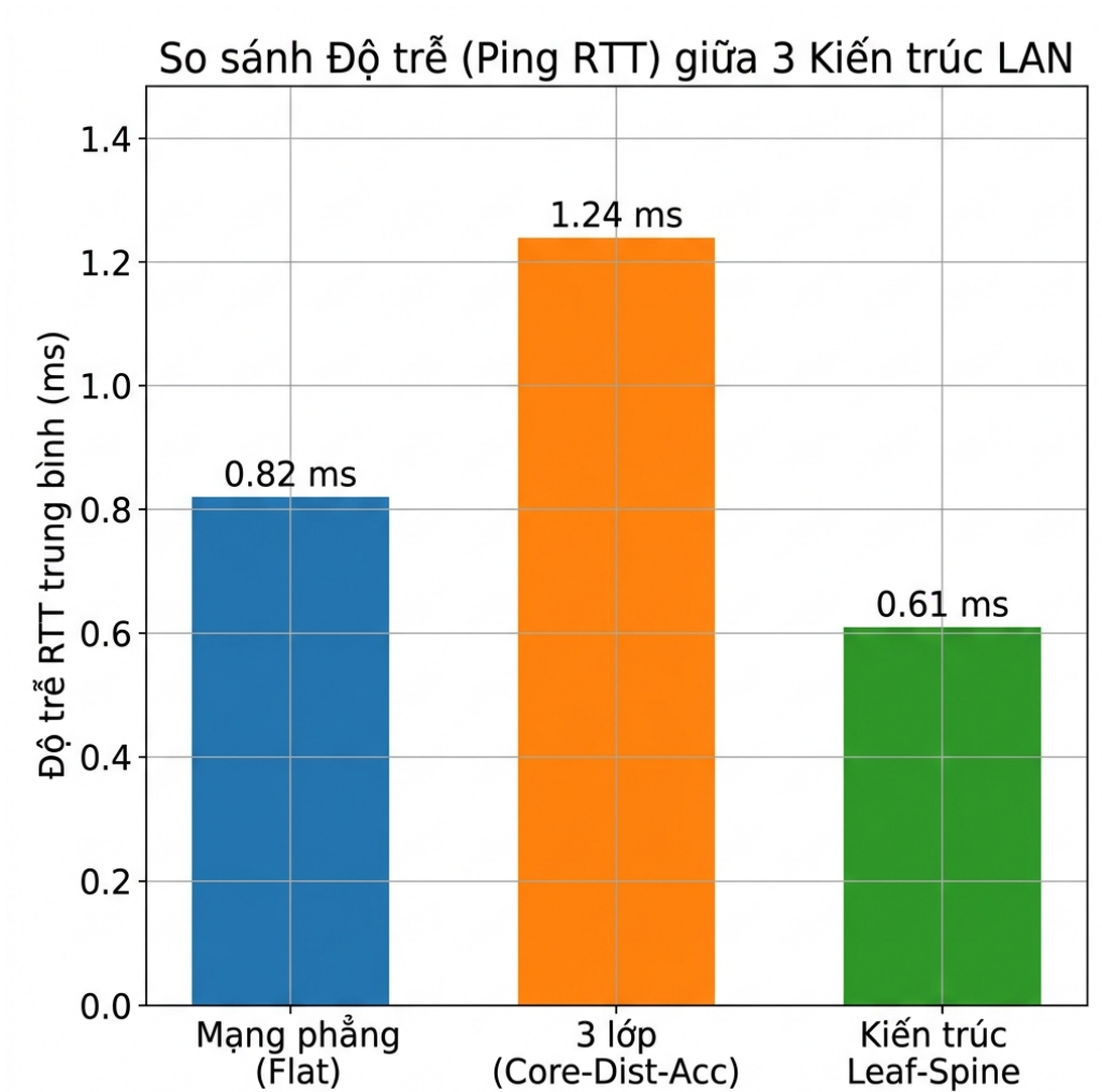
Hình 5.3: Delay (Ping RTT trung bình, ms) theo từng kịch bản đo lường
