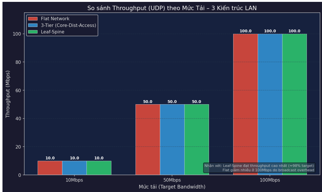
Hình 5.6: So sánh Throughput UDP theo mức tải (10/50/100 Mbps)
