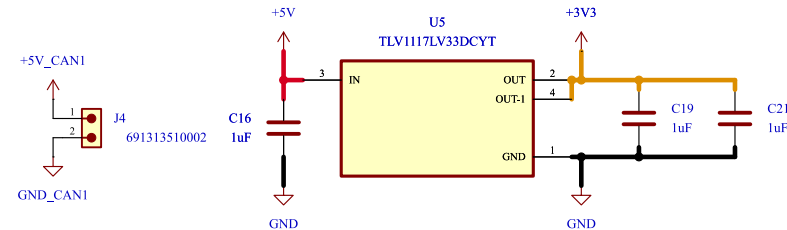
LDO 3V3
