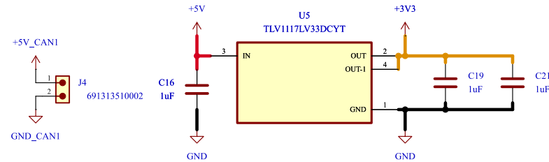
LDO 3V3
