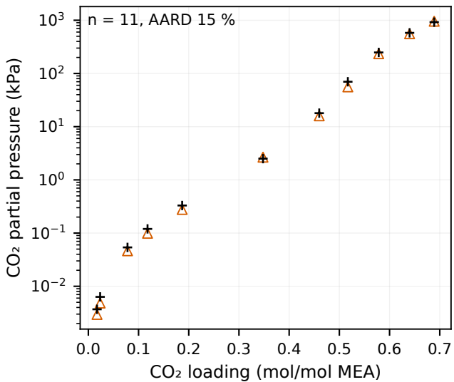
80 °C · prediction
