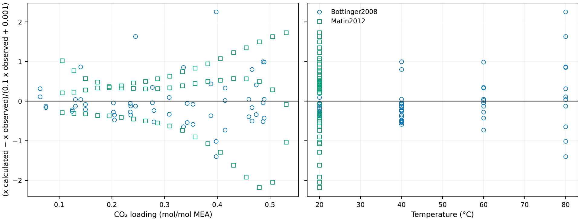
heat F1 species · Matin pool shown separately
