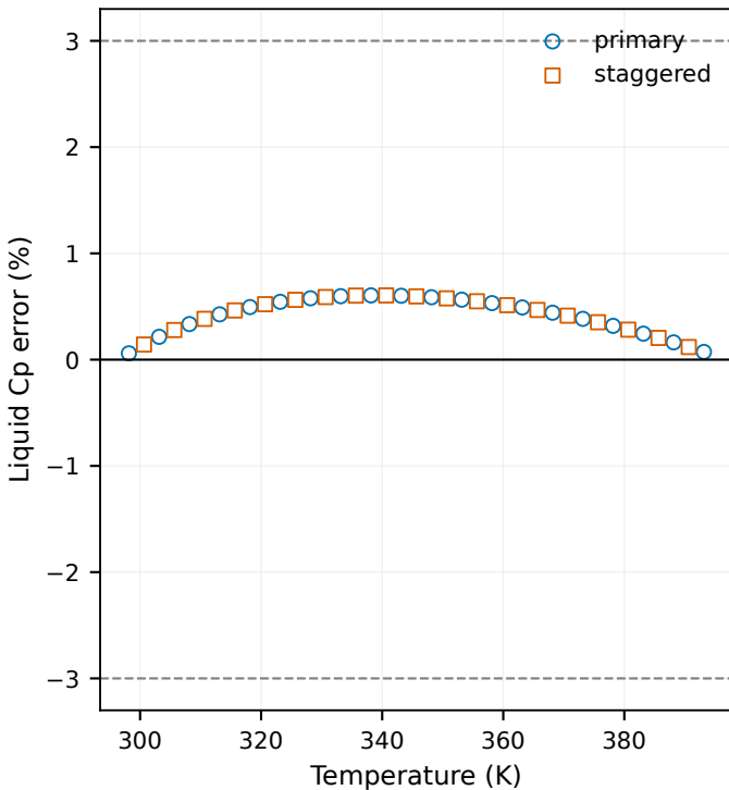
Cp at 0.300 MPa; \pm 3\% limit
