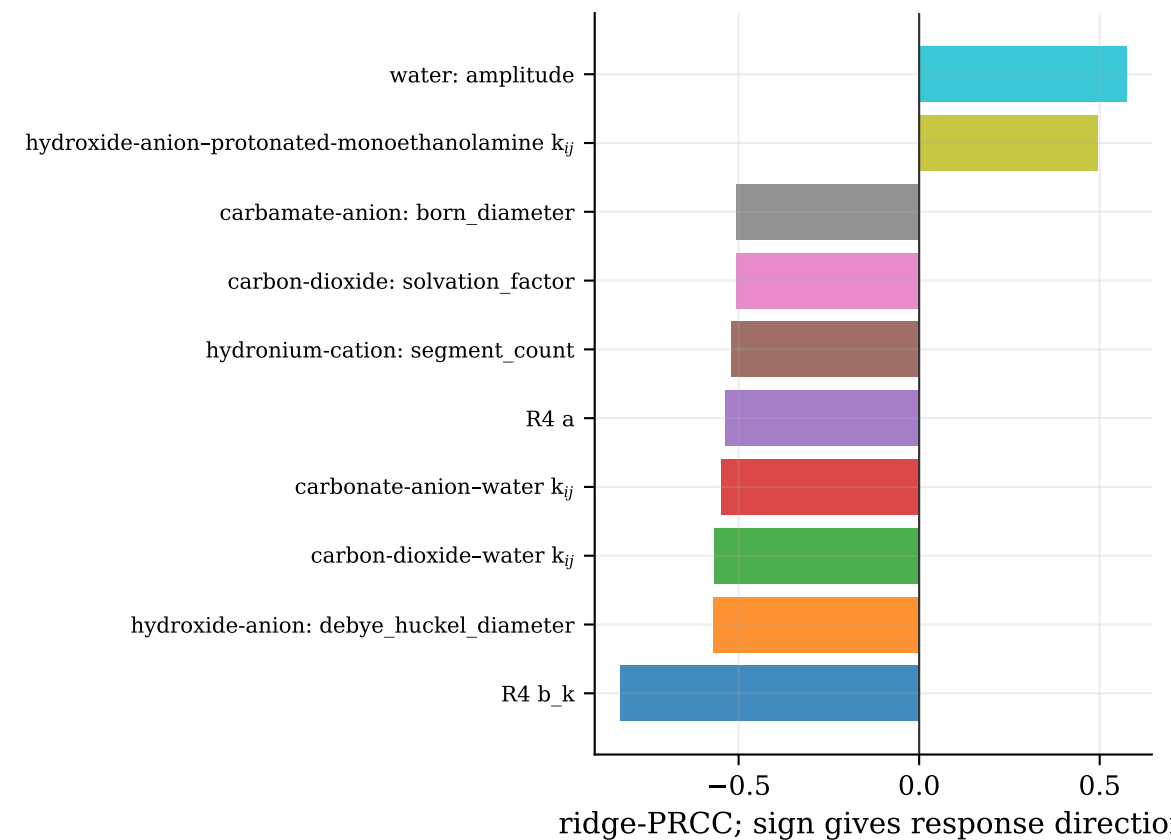
\log_{10} n_{MEA COO^-}
