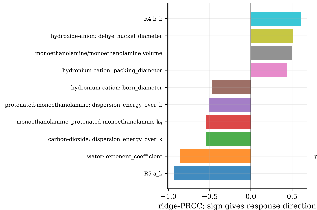
\log_{10} n_{MEA H^+}
