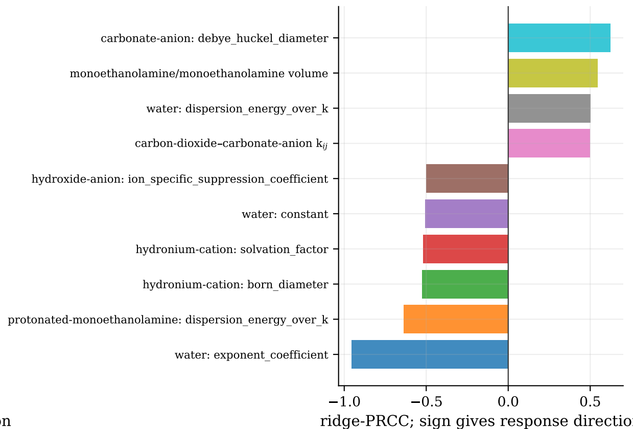
\log_{10} n_{MEA COO^-}
