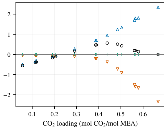
(d) F3 – F1 decomposition, 60 °C
