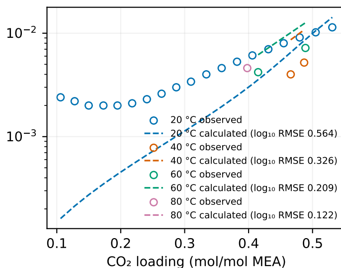
HCO3-
