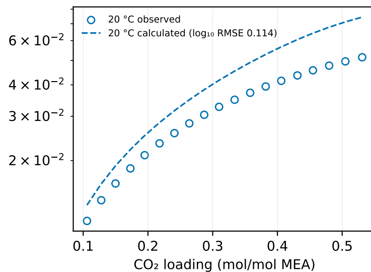
HCO3-
