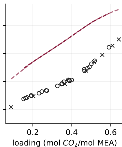
M5: full DD + QQ + DQ RMSE = 2.746
