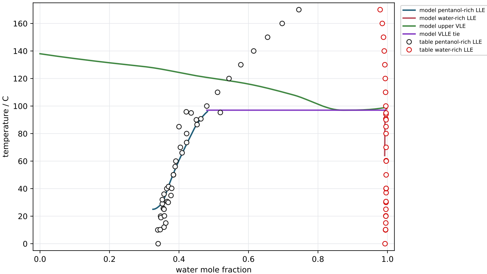
Gross 2002 Fig. 10: water/1-pentanol LLE
