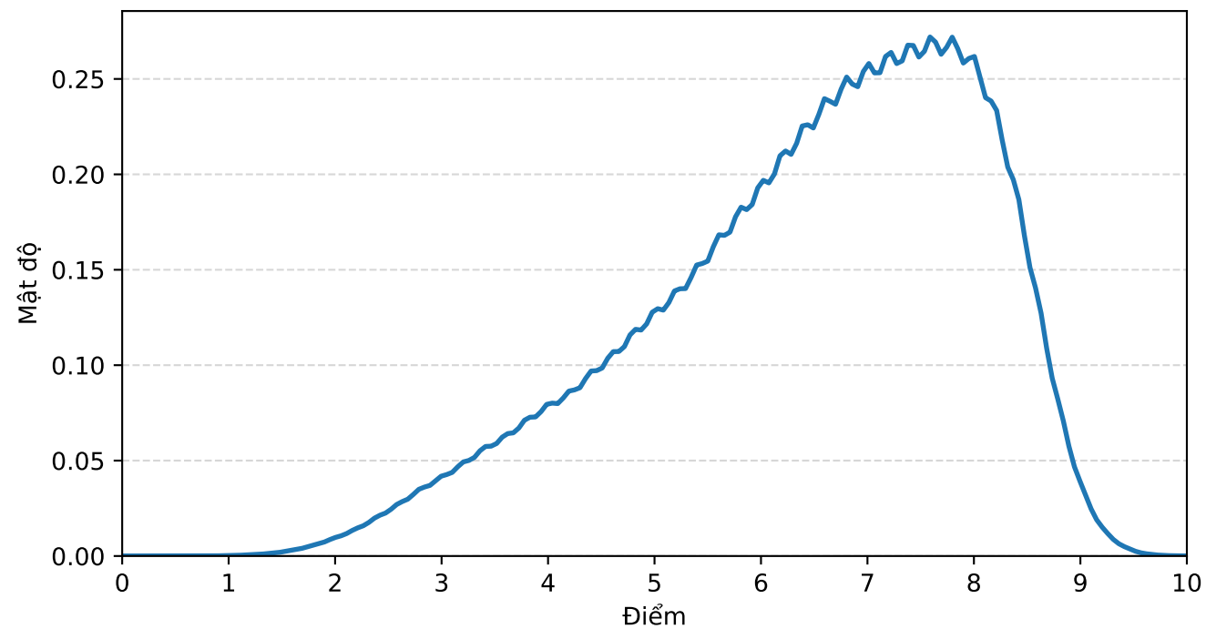
KDE điểm môn toán - năm 2024
