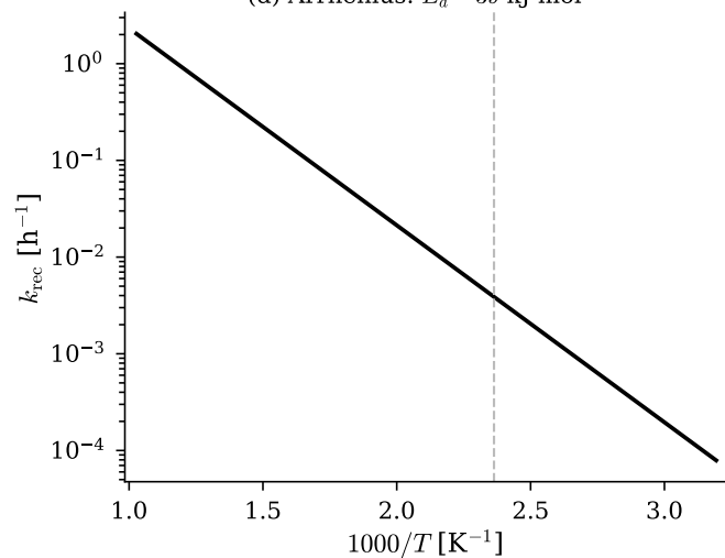
(d) Arrhenius: E_a = 39 \text{ kJ mol}^{-1}
