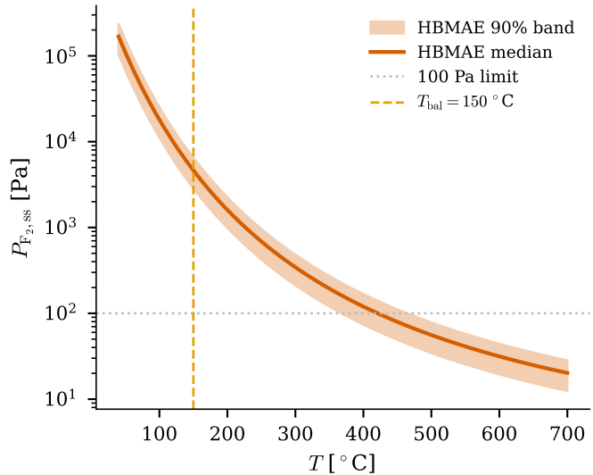
(b) P(F_2)_{ss} vs T
