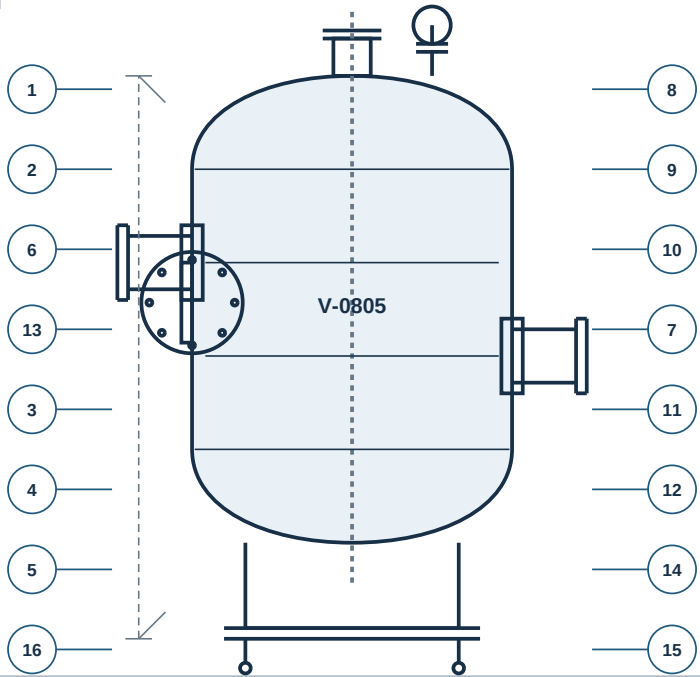
ELEVATION | O/A HEIGHT 3200
