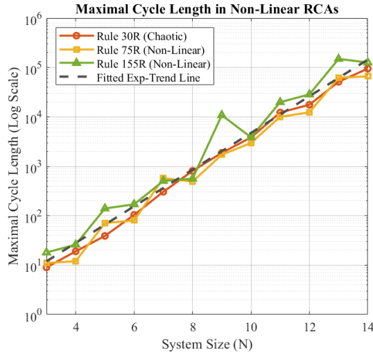
FIG. 3. 非线性混沌规则（30R、75R、155R）最大周期随尺寸 N 的联合对比图（纵轴为对数轴）。深色虚线为通过最小二乘法回归拟合出的平均指数增长趋势线。
