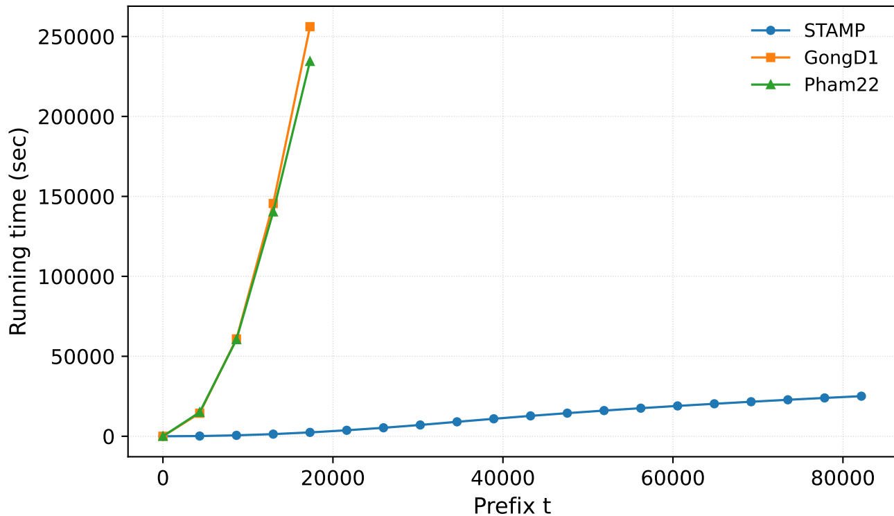
Slashdot.bin (n=82168, K=3, B=16433)
