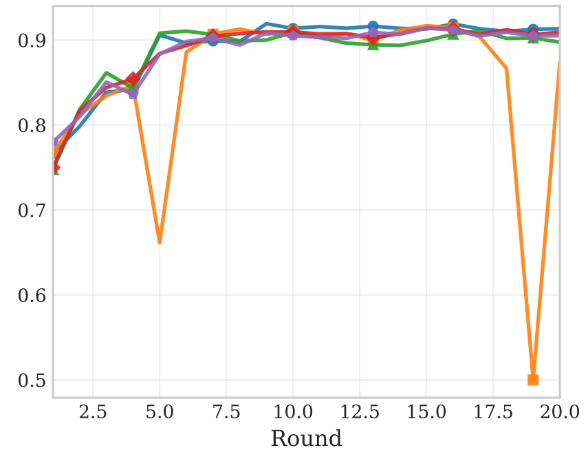
AUC-ROC - Scenario C
