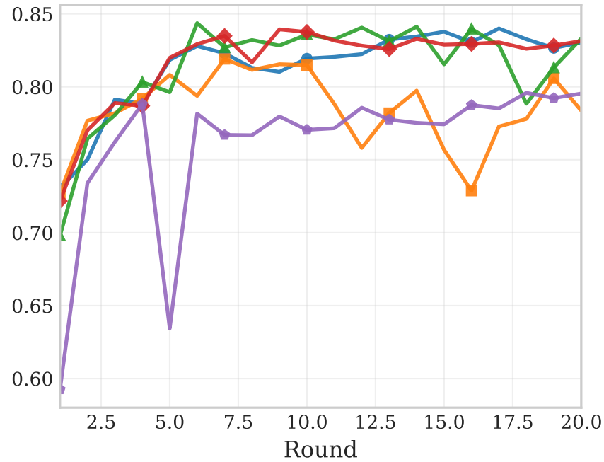
AUC-ROC - Scenario B
