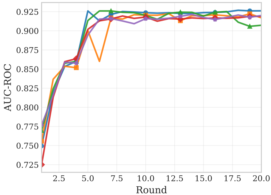
AUC-ROC - Scenario A
