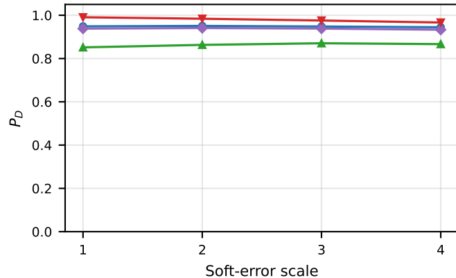
error sigma
