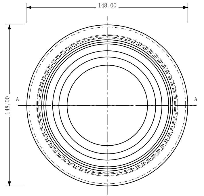
右向端视图（独立标注）
