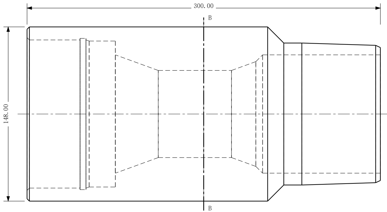
主视图（沿图纸 Z 方向）
