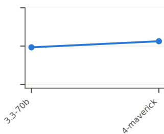
Llama
