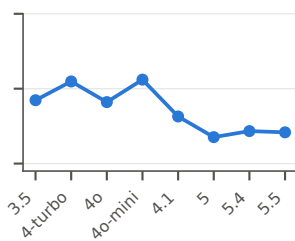
GPT
