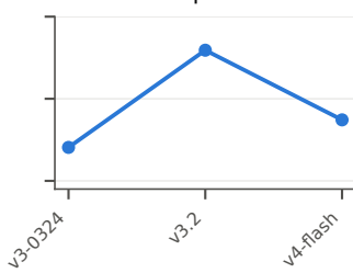
DeepSeek
