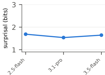
Gemini
