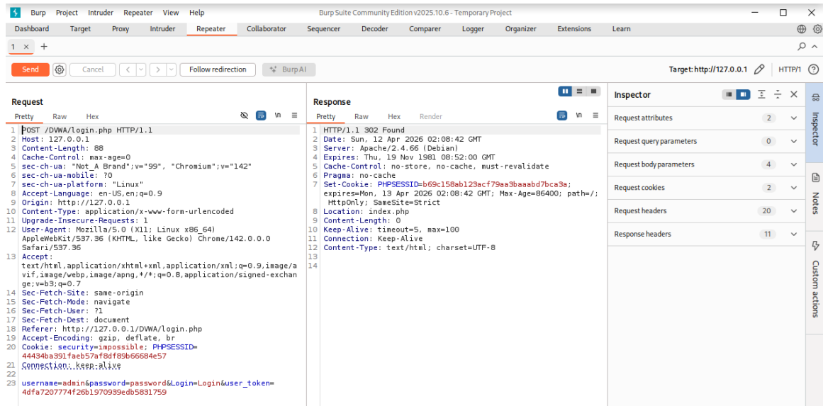
Рисунок 4.4: Информация по входу на сайт DVWA
