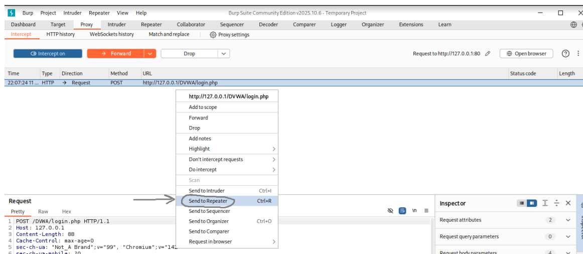
Рисунок 4.3: Окно Burp Suite и нажатие на «Send to Repeater»
