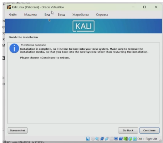
Рисунок 20: Перезагрузка
