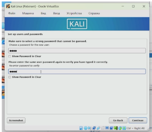
Рисунок 12: Пароль
