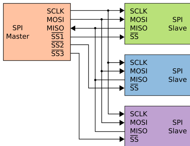
Рис. 7.1 – Топология SPI с общими линиями данных и отдельными сигналами выбора ведомых устройств
