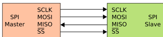
Рис. 7.2 – Подключение одного SPI-устройства к Lichee RV Dock
