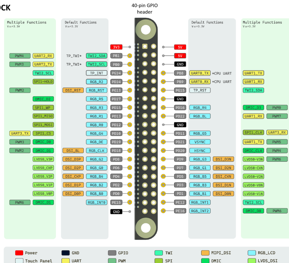
Рис. 3.5 – Распиновка Lichee RV Dock — SPI на альтернативных выводах
