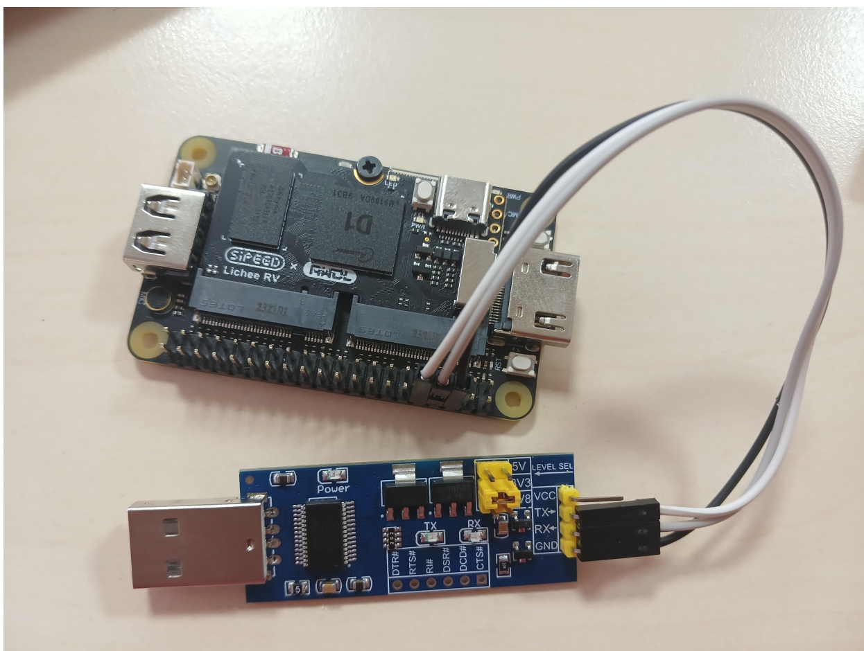
Рис. 1.2 – UART-преобразователь
