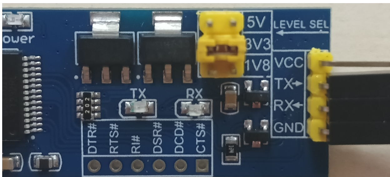
Рис. 1.1 – Джампер
