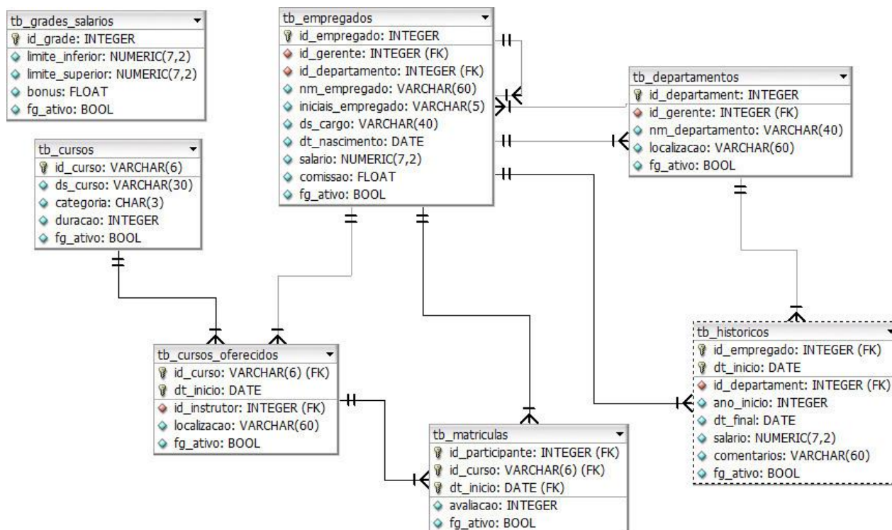
Figura 2 – Esquema de Banco de Dados Relacional Hipotético
