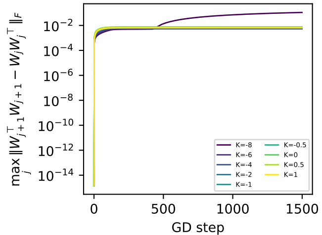
(d) \delta -balancedness
