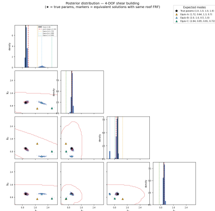
図 2 4 自由度せん断建物の事後分布散布図
