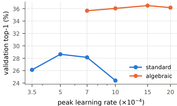
ViT-S/8, 64 px, 4 epochs
