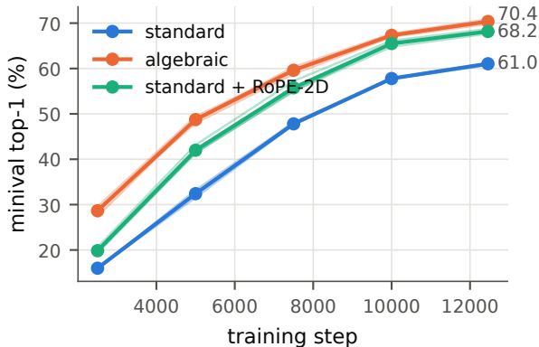
ViT-B/16, 224 px, 2.5B tokens
