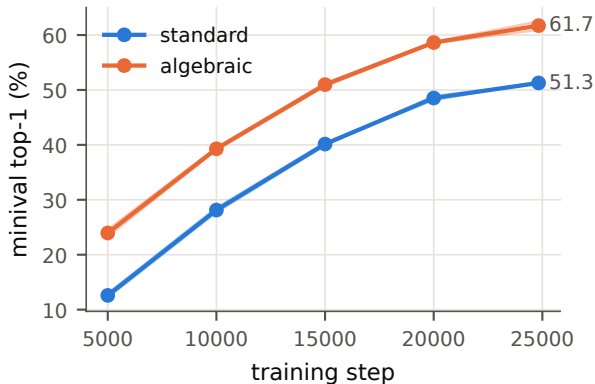
ViT-S/4, 64 px, 10 epochs
