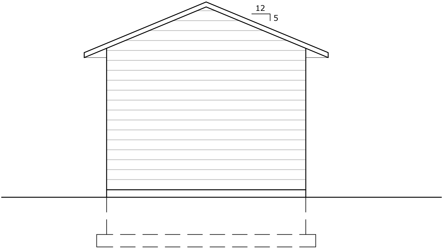
BACK ELEVATION SCALE: 1/4" = 1'-0"
