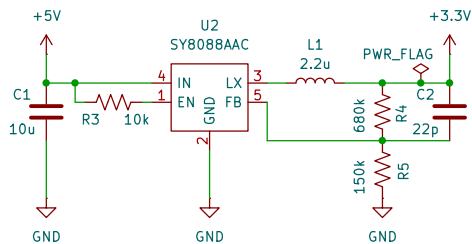
レギュレータ 5V → 3.3V
