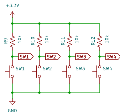
タクトスイッチ (4つ)
