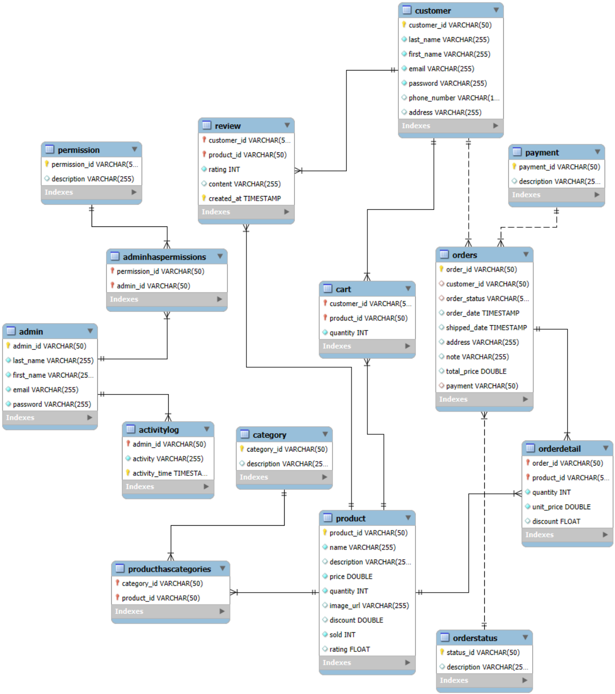
Hình 3.17 Mô hình RDM
