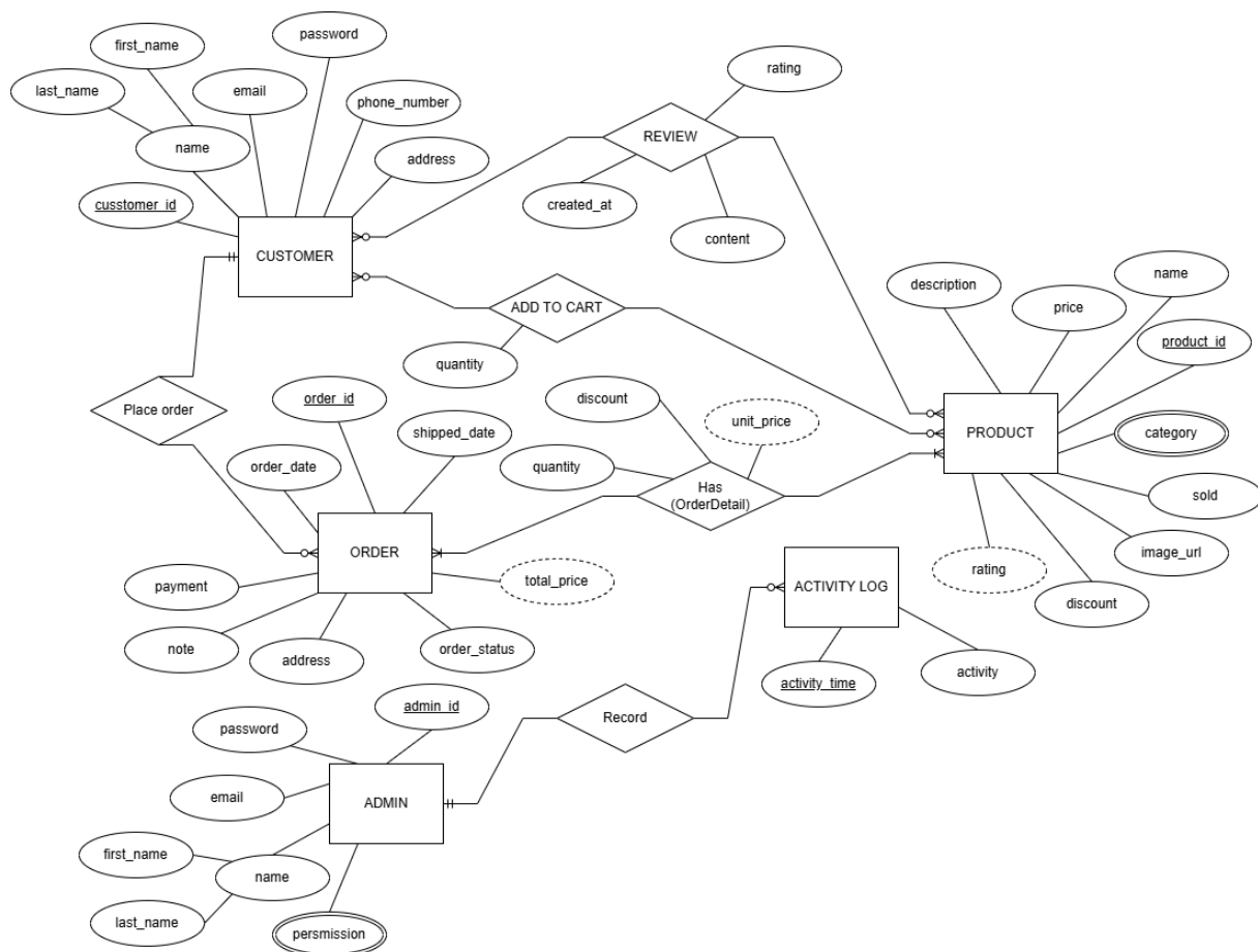
Hình 3.17 Mô hình ERD
