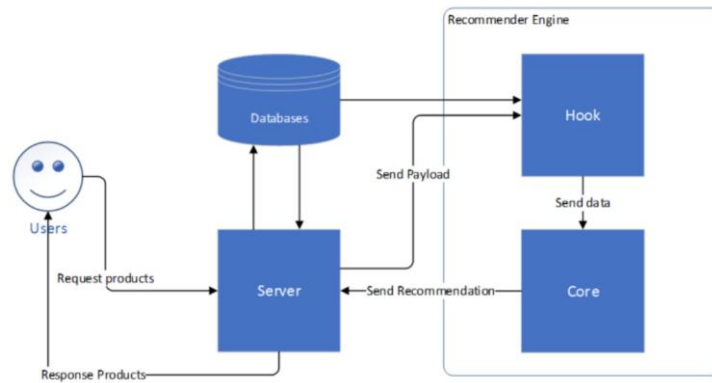
Hình 2.3 Kiến trúc hệ thống gợi ý [7]
