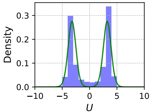
DM: y = 0 \cdot \mathbf{1}_{10}
