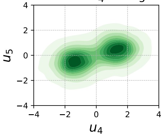
True: u_4 vs u_5
