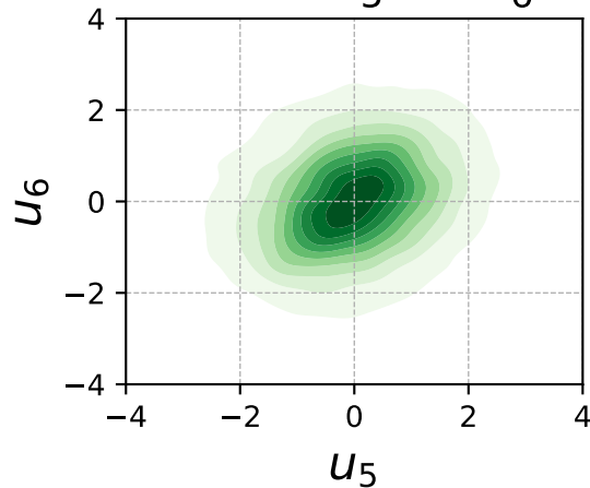
True: u_5 vs u_6
