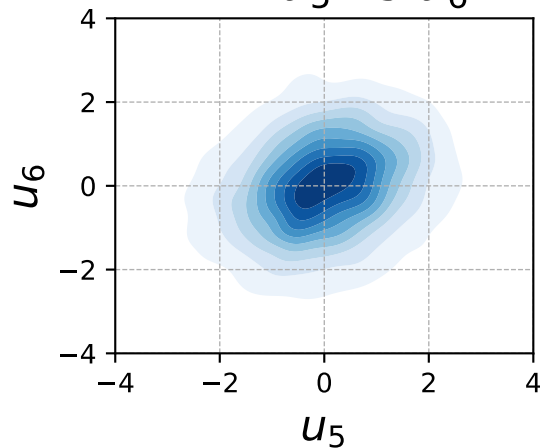
NN: u_5 vs u_6
