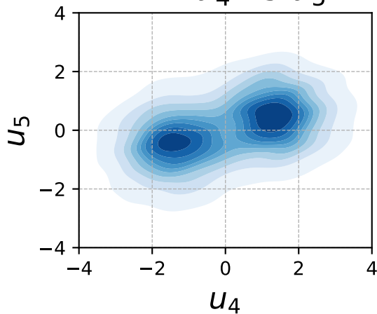
NN: u_4 vs u_5
