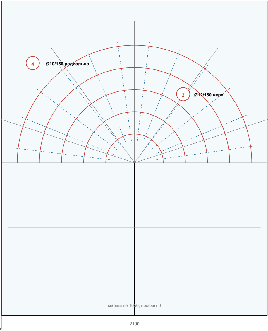
ПЛАН ЗАБЕЖНОГО УЗЛА
